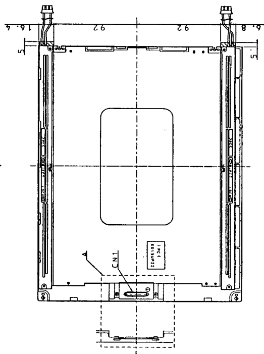
Fig1 LQ121S1DG11 OUTLINE DEMENSIONS
